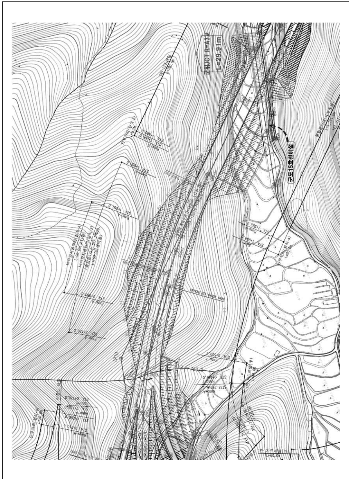
【그림 34.1.4】 평면도
